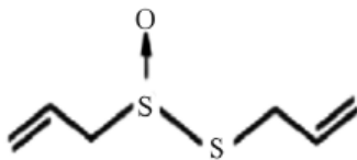
Allicina
