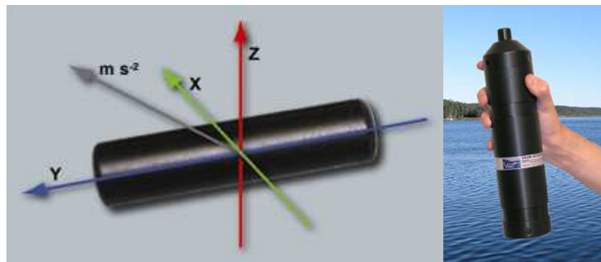
Figura WP3. 8. schema del funzionamento dell'accelerometro V9A della Vemco (sulla sinistra); immagine del ricevitore VR2W della Vemco (sulla destra).
