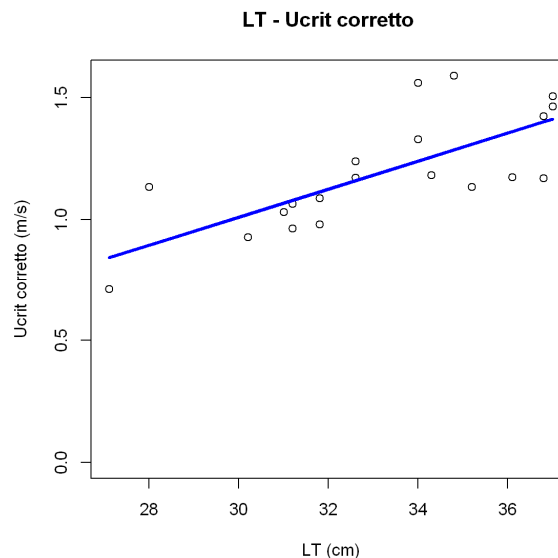
Figura WP3.14 Regressione lineare tra lunghezza totale e U_{crit} corretto ( n = 20 , p -value=0.00024).
