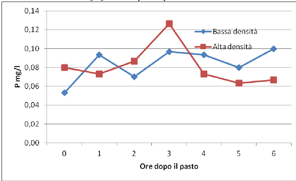
WP4.2 – Andamento del fosforo in impianto produttivo alle due densità.
