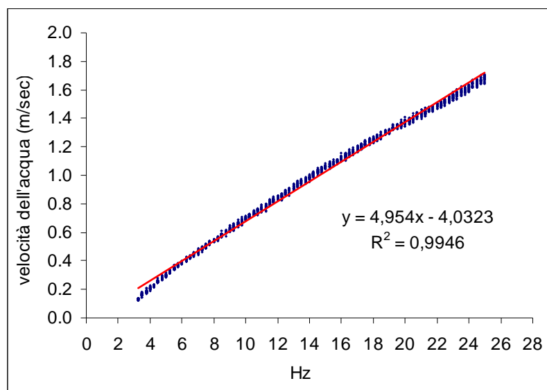
Figura WP3.2 Calibrazione della camera di Blažka: relazione tra frequenza e velocità dell'acqua.
