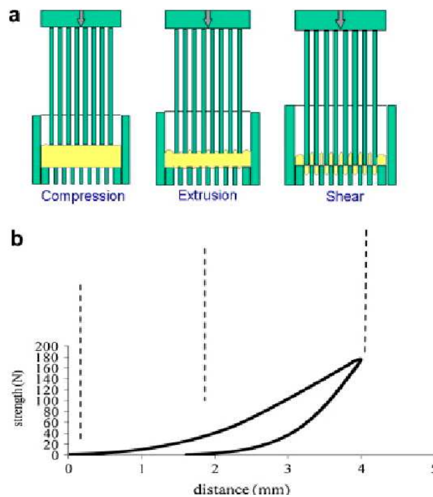
Figura WP6.4. Schema illustrante il principio di funzionamento della Kramer shear-press (a), con il corrispondente andamento della forza coinvolta vs la distanza percorsa dal probe durante l'analisi (b).
