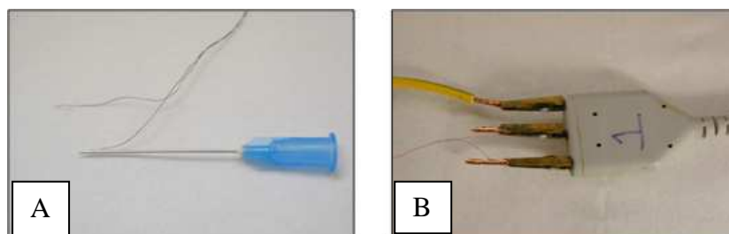
Figura WP3.7 Elettrodi fine wire prima del posizionamento intramuscolo; B: Collegamento degli elettrodi e della messa a terra ad uno dei terminali.
