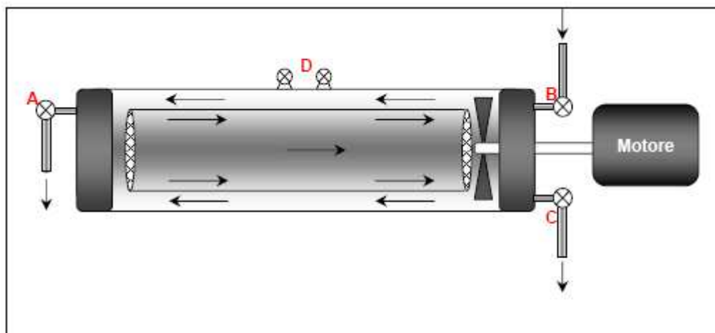
Figura WP3.1 Rappresentazione schematica della camera di Blažka. A,C: valvole di scarico; B: valvola di carico; D: valvole per lo svuotamento dell'aria ed inserimento dei sensori.
