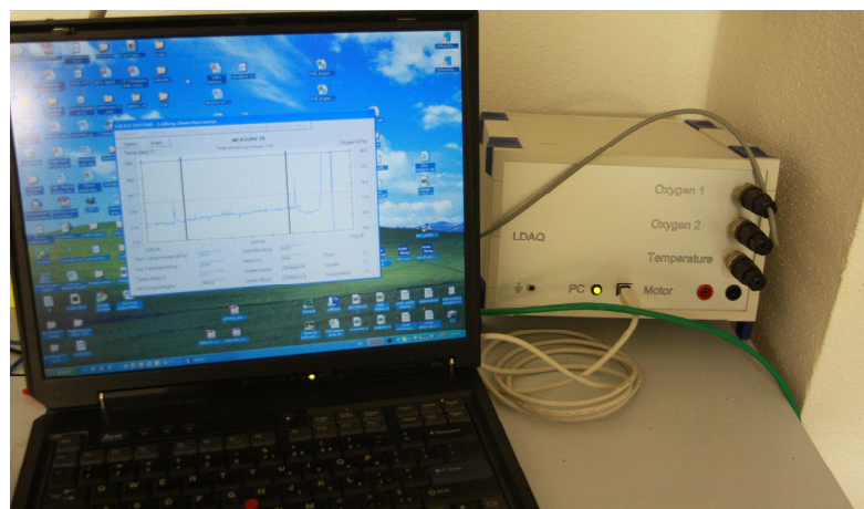
Figura WP3.3 Respirometro DAQ-1 (Loligo system) connesso al PC per la raccolta dei dati sperimentali.
